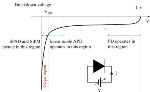
图 23: 不同光电二极管伏安特性曲线电压工作区间示意图
