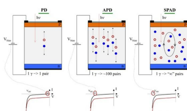
图 24: 不同探测器微观原理示意图
