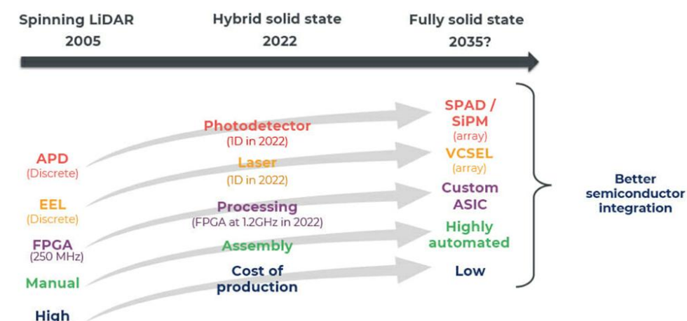
图 28: 2005-2035 年车载激光雷达技术路线图
