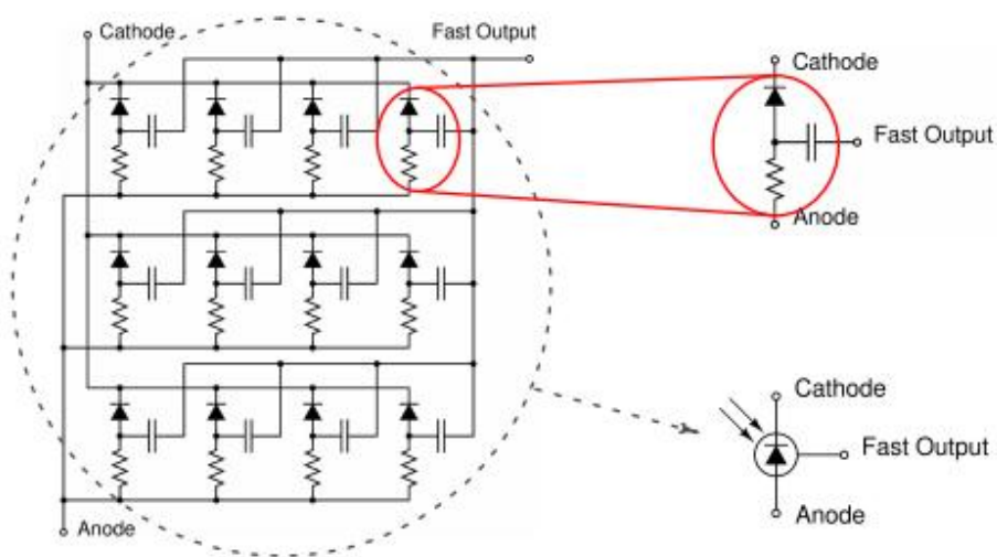
图 25: SiPM 简化电路结构示意图
