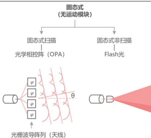
图 16: 固态式激光雷达原理示意图
