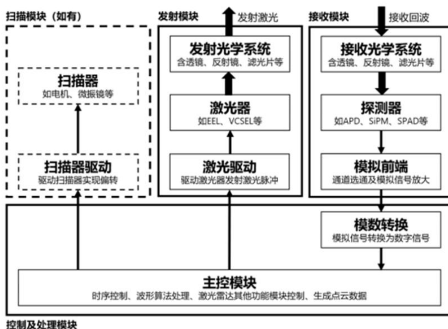
图7：激光雷达核心模块示意图
