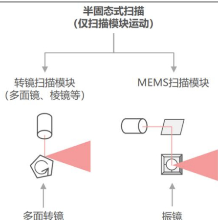
图 14: 半固态式激光雷达原理示意图
