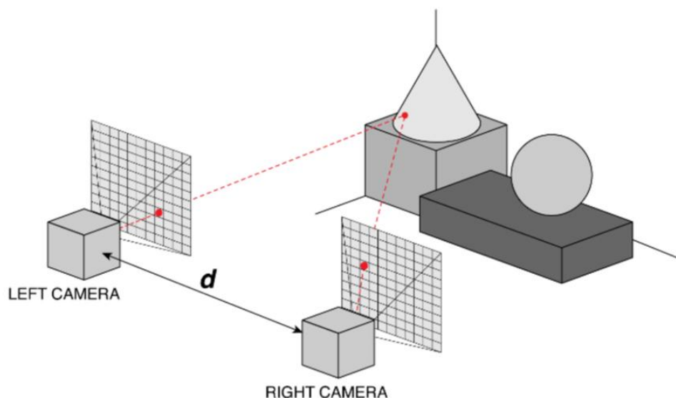
图20: 三角测距法原理示意图
