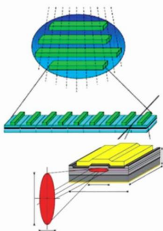
图8：EEL 芯片示意图
