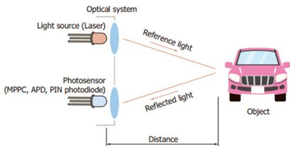
图5: 激光雷达测距原理示意图
