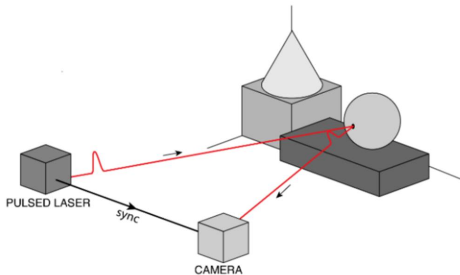
图21: ToF 测距法原理示意图
