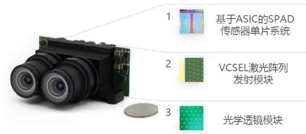
图4: Ouster Flash 激光雷达示意图
