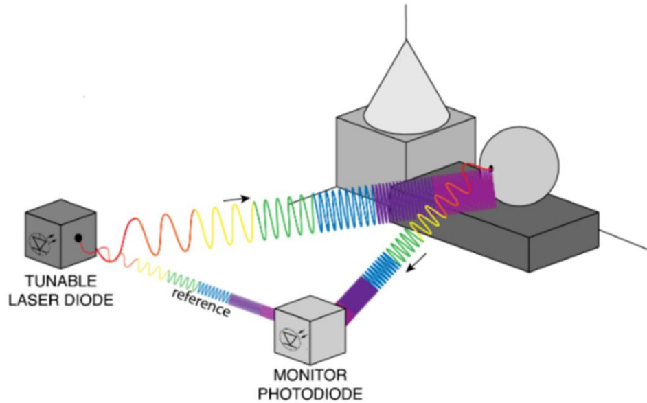
图 22: FMCW 测距法原理示意图
