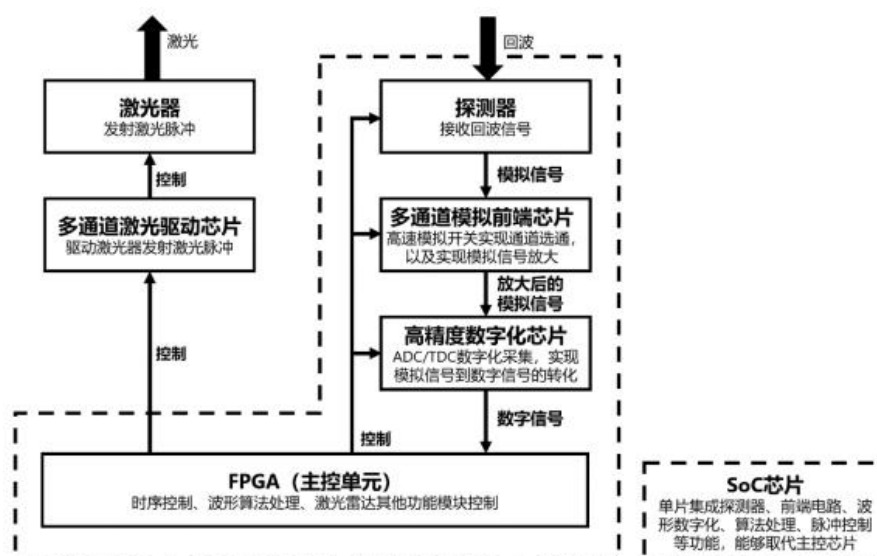
图 27: 激光雷达专用芯片及功能模块示意图
