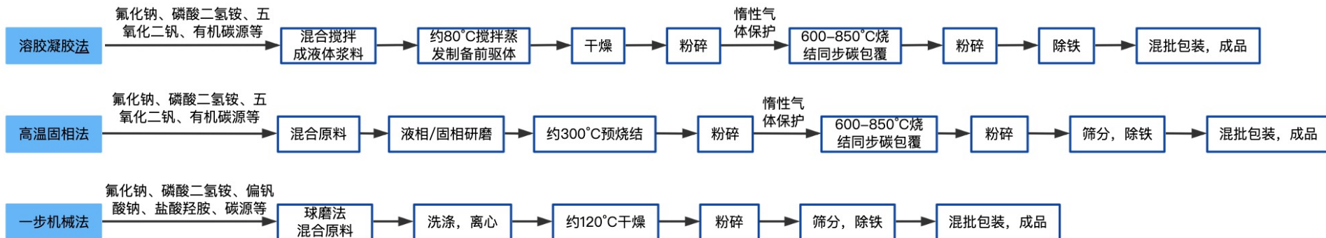
图表：聚阴离子制备工艺路线
