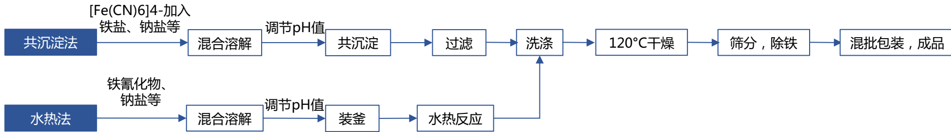
图表：普鲁士蓝/白制备工艺图
