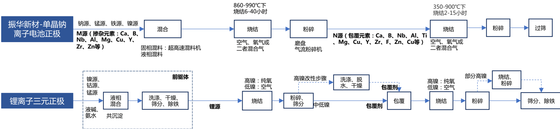
图表：层状氧化物工艺流程与三元正极工艺流程对比
