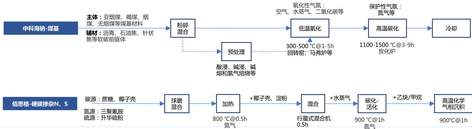
图表：部分钠离子电池负极加工流程
