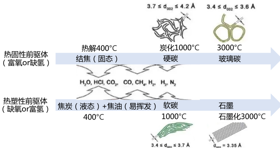
图表：硬碳与软碳前驱体炭化原理
