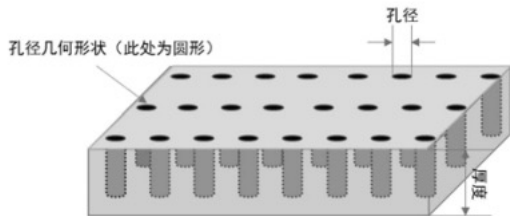
图表：一种抑制钠枝晶的多孔铝集流体
