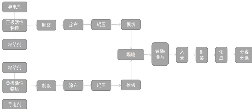
图表：钠离子电池生产工序
