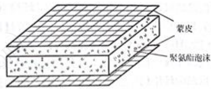
图 3-13 泡沫夹心结构复合材料
