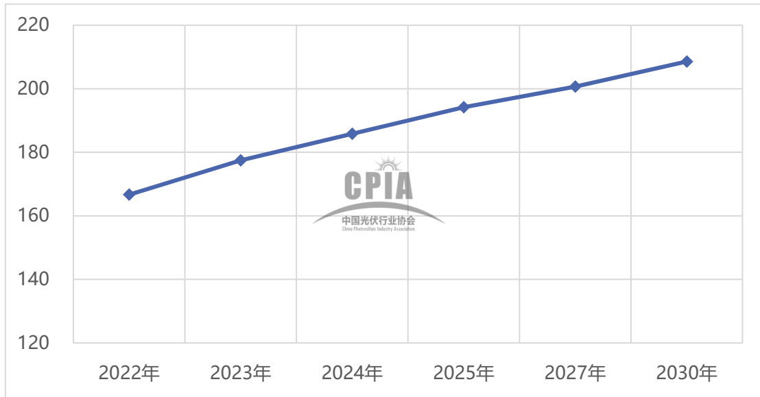
图 42 2022-2030 年 p 型电池片发射极方块电阻变化趋势 (单位: ohm/cm²)
