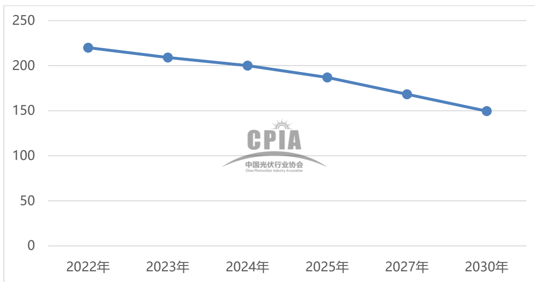
图 83 2022-2030 年锂电储能单位装机占项目用地变化趋势 (单位: m 2 /MW)
